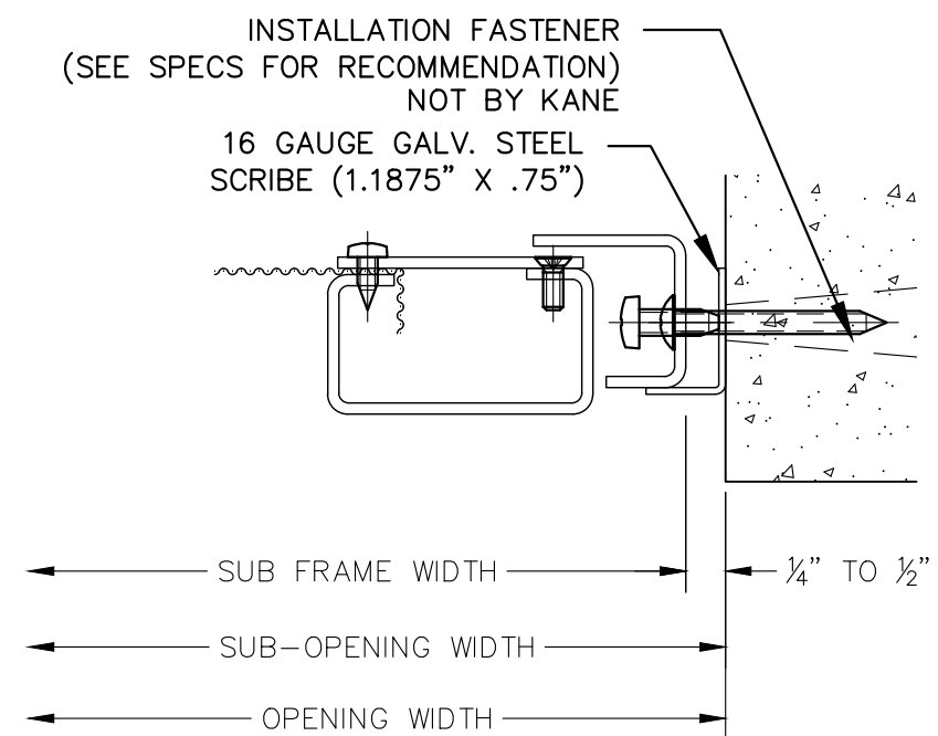
4 RIGHT JAMB SCALE: 6"=1'-0"
